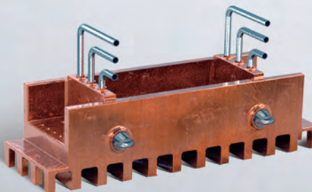
Élément: Fabriqué en cuivre moulé à haute conductivité, au-dessus de 77% IACS
